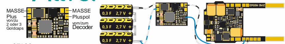
STACO1 10 x 7.3 x 2 mm (CAD 2:1 vergrößert)
