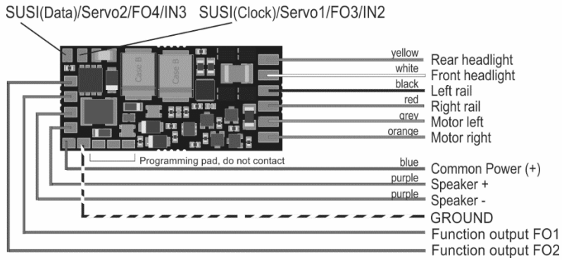
MS490N, MS490L Top side, NEM 651 . SOUND
